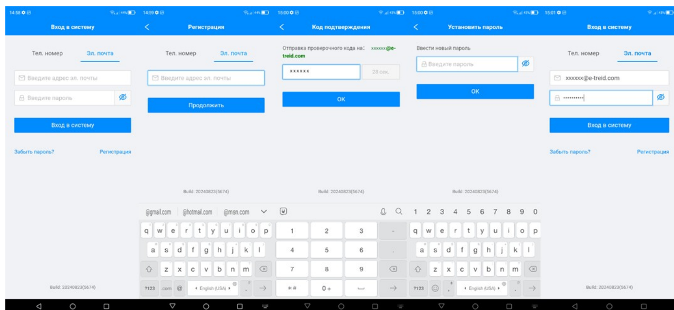
Android
